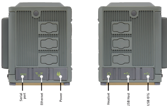
Рисунок 3. Порты приемника
