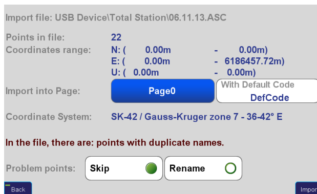
Рисунок 103. Импорт точек
