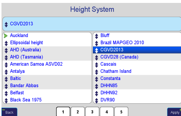
Рисунок 29. Система высот
