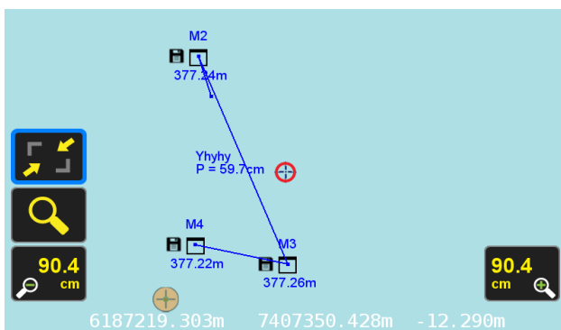
Рисунок 61. Съемка полилинии
