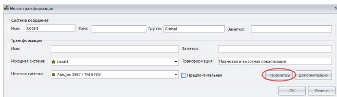
Рисунок 41. Параметры
