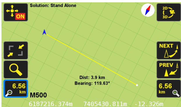
Рисунок 74. Режим карты
