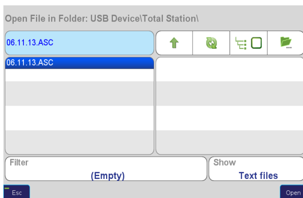
Рисунок 101. Выбор файла
