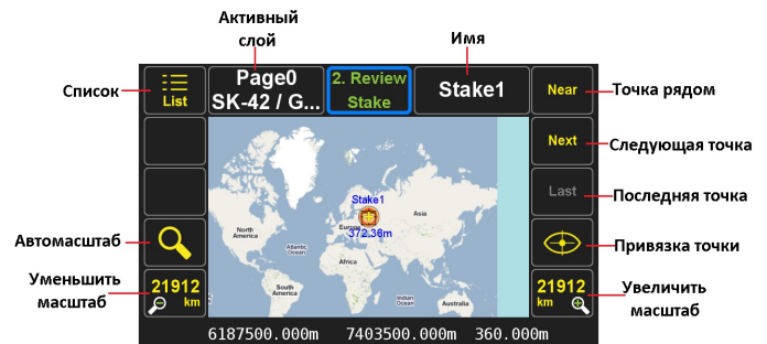
Рисунок 71. Экран Review
