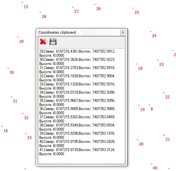
Рисунок 96. Coordinates clipboard
