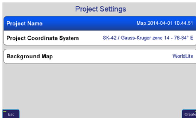
Рисунок 10. Project Settings
