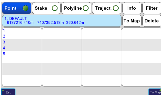
Рисунок 59. Список объектов
